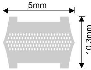
Perfil AA
